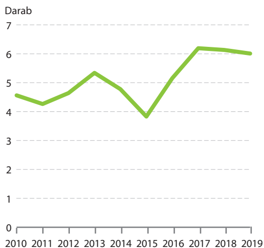
7.4. ábra A tíz kilométer ivóvízvezetékre jutó csőtörések számának alakulása
